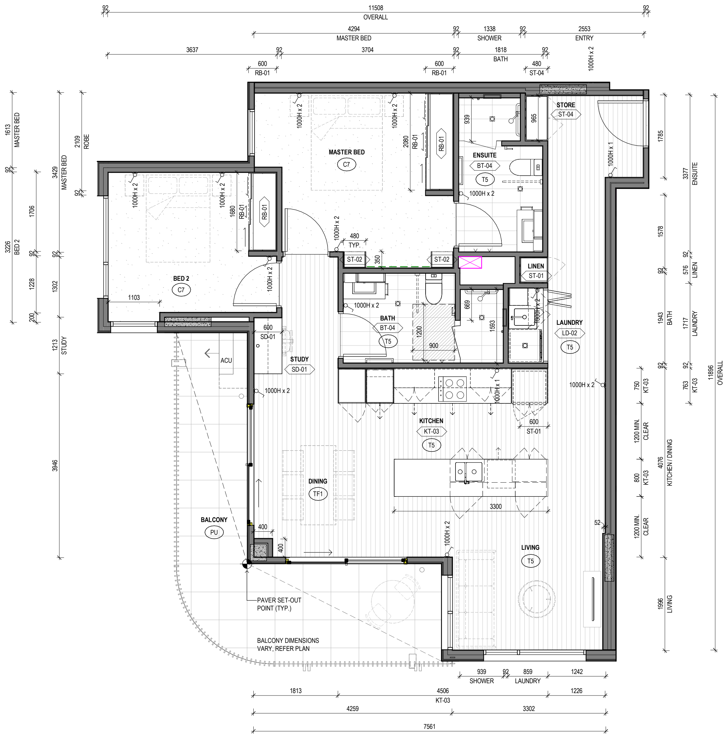
1 ILA Type 4 Scale 1 : 50
